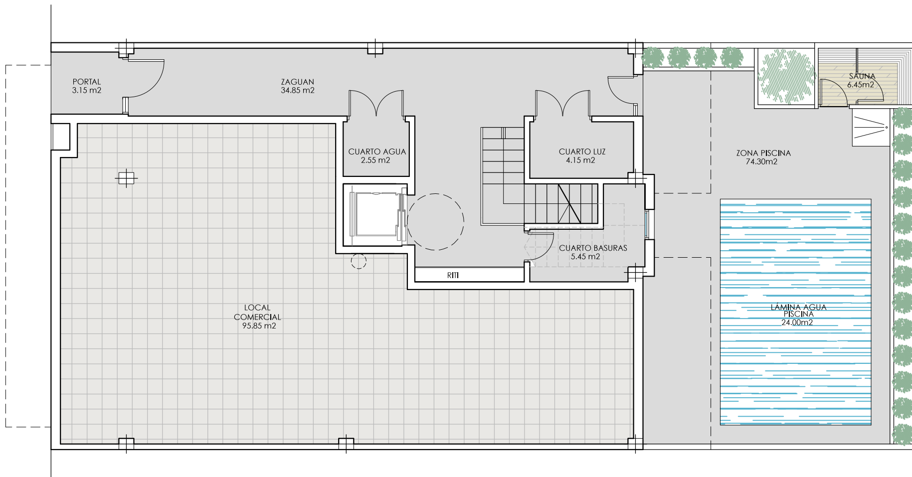
Planta Baja
