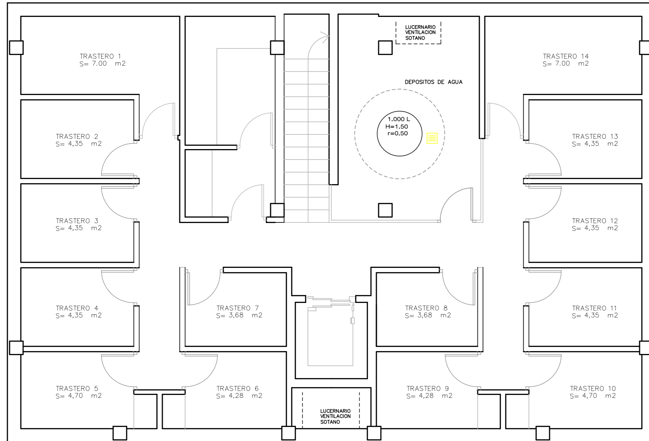
PLANTA SOTANO
